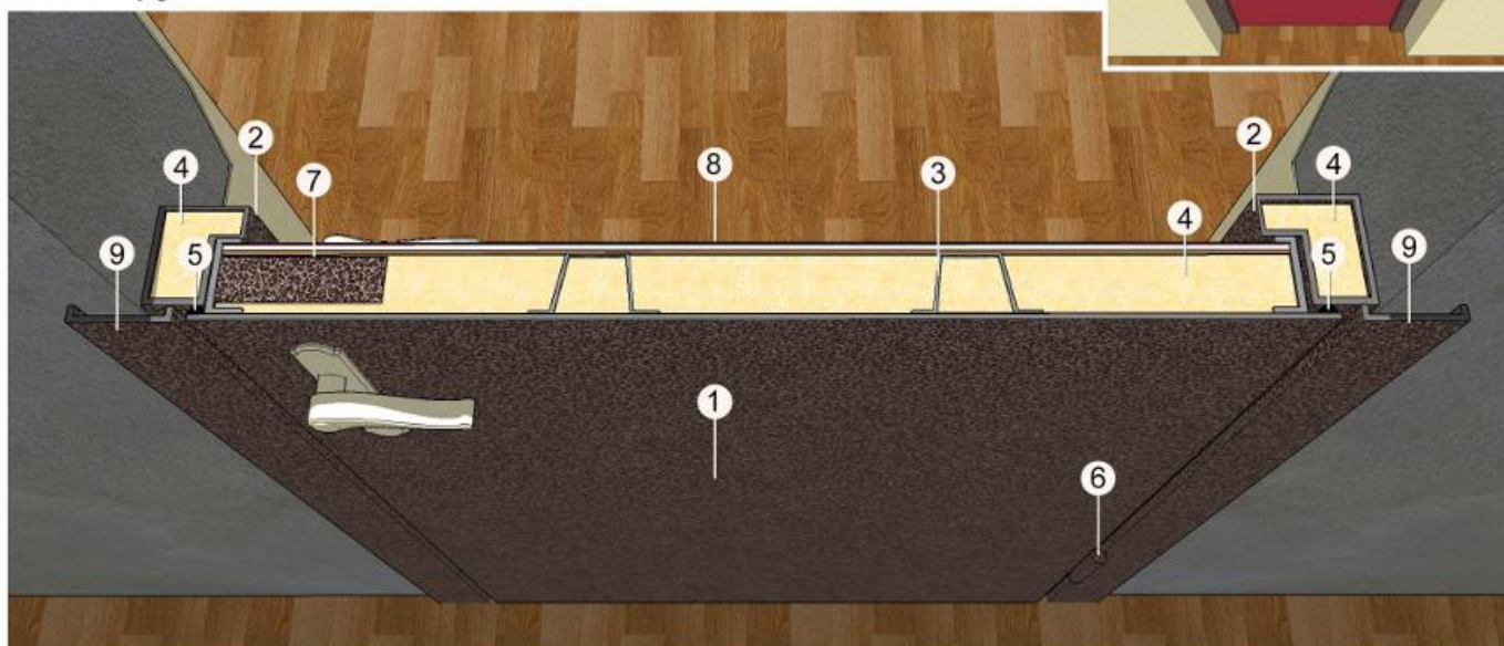
Вид снаружи
