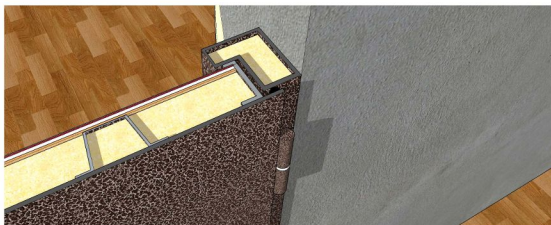
Установка с наличником
